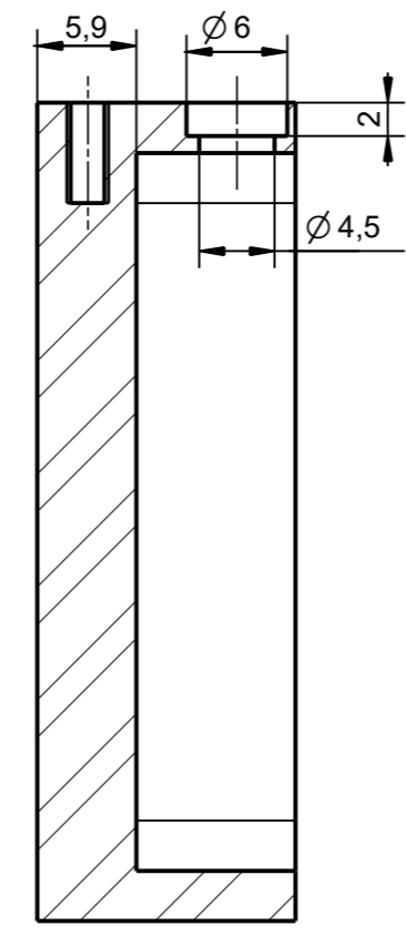
Schnitt A-A
